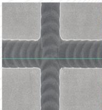
ITO刻线 ( 显微放大 )
